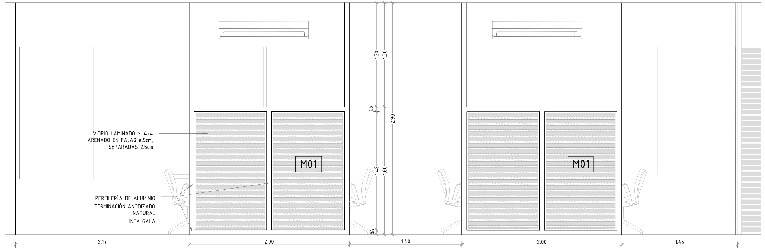
ALAZADO MAMPARAS M01 ESC 1.25
