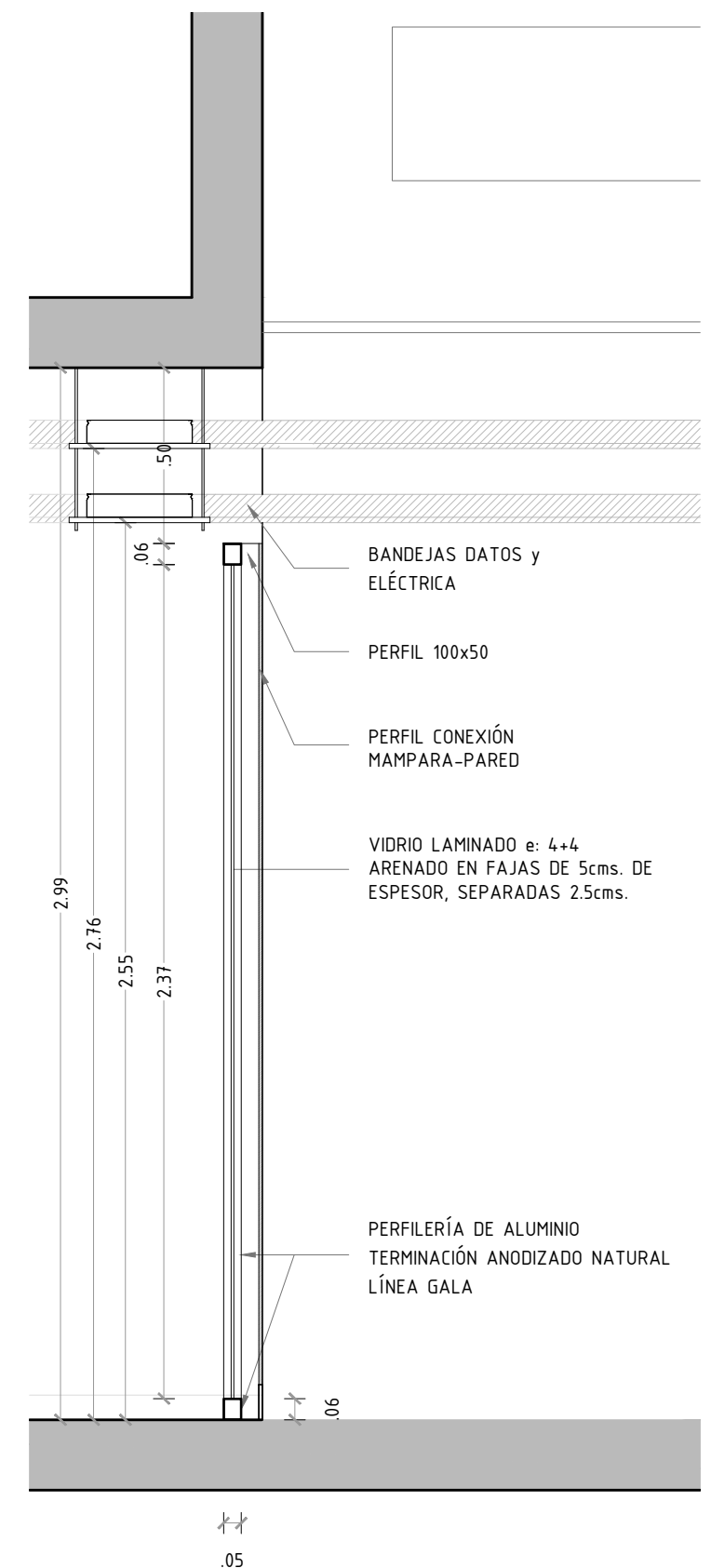
CORTE M04 ESC 1.20
