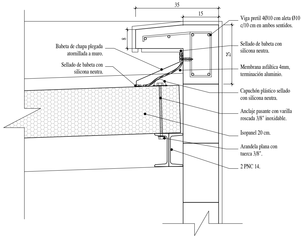
Detalle Punto alto isopanel esc. 1:10
