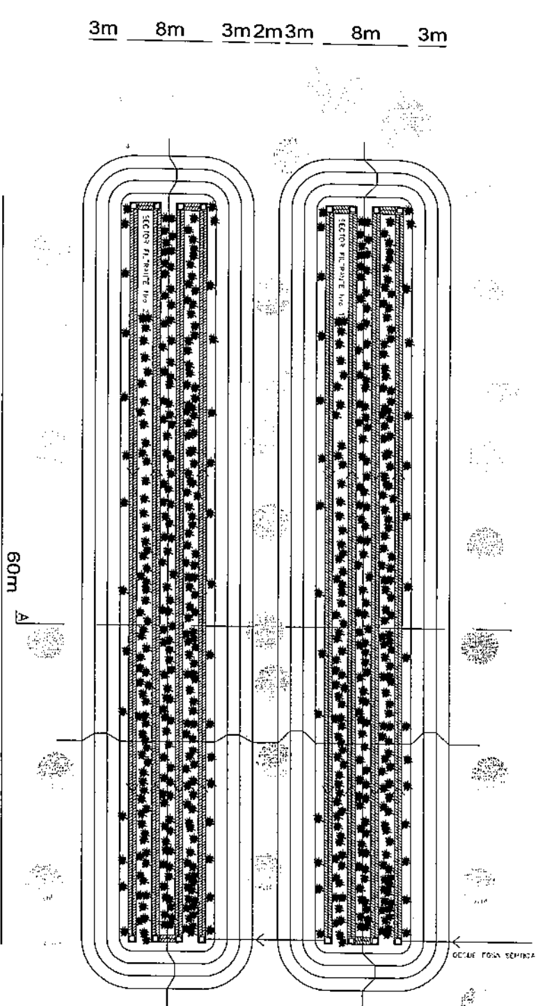
PLANTA SISTEMA DE INFILTRACIÓN SUBSUPERFICIAL esc 1:200
