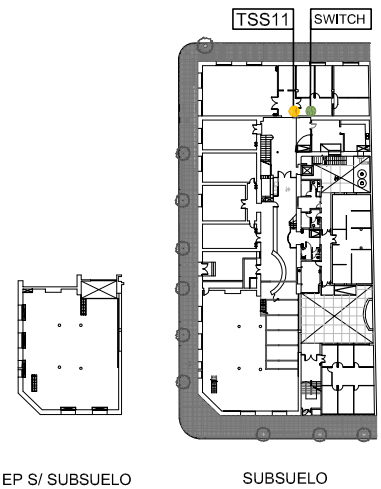
SUBSUELO
