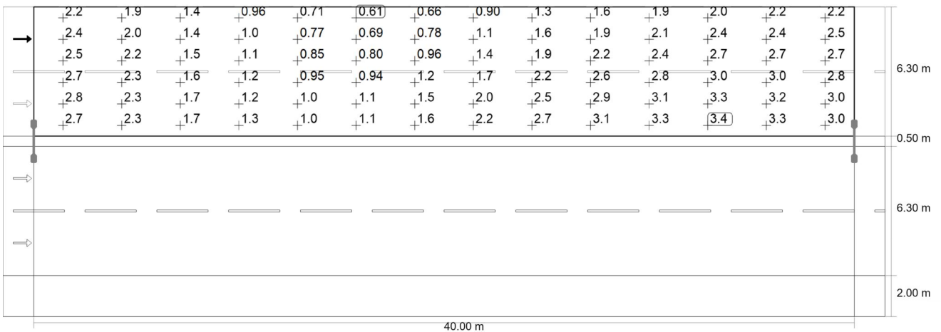
Observador 2: Luminancia para una instalación nueva [cd/m²] (Sistema de valores)
