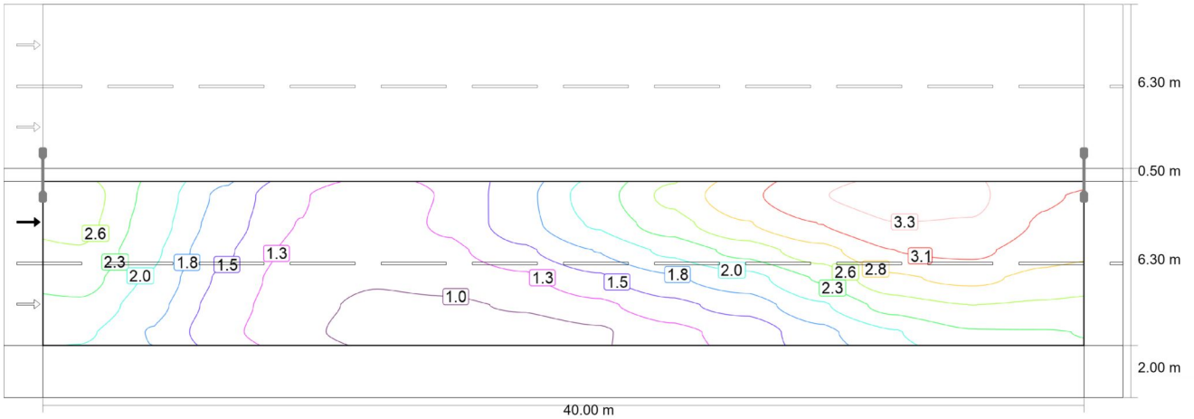
Observador 2: Luminancia para una instalación nueva [cd/m 2 ] (Líneas Isolux)
