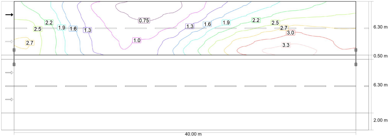
Observador 2: Luminancia para una instalación nueva [cd/m²] (Líneas Isolux)
