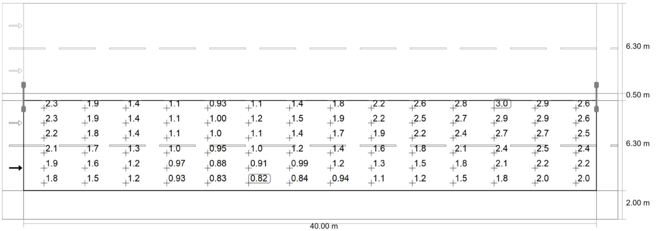
Observador 1: Valor de mantenimiento luminancia en calzada seca [cd/m 2 ] (Sistema de valores)
