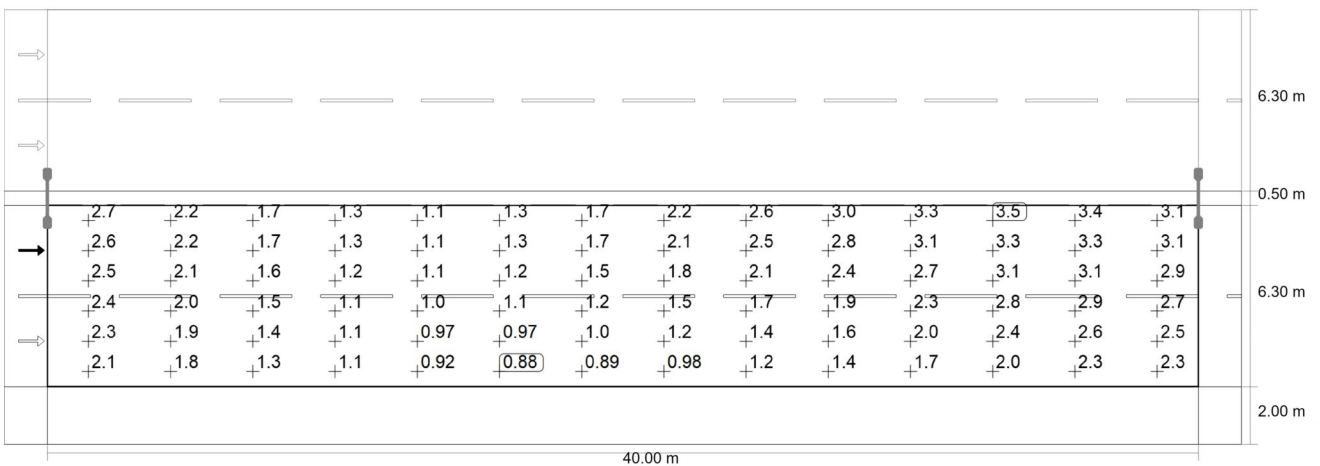
Observador 2: Luminancia para una instalación nueva [cd/m 2 ] (Sistema de valores)
