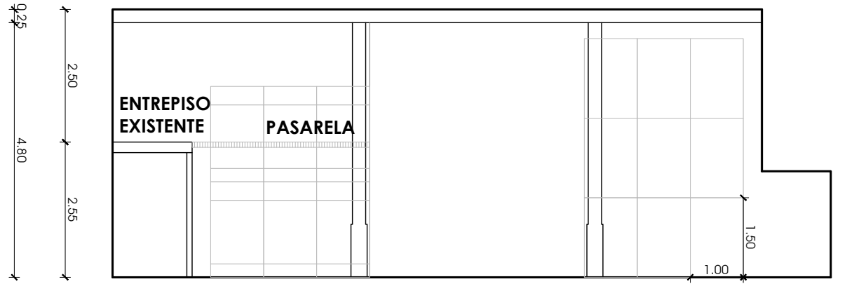
CORTE BB
